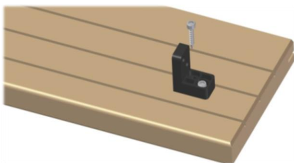
Figur 6: Skruva fast den tjockaste delen av ändclipset på altanbrädan – ett clip för varje regel.
