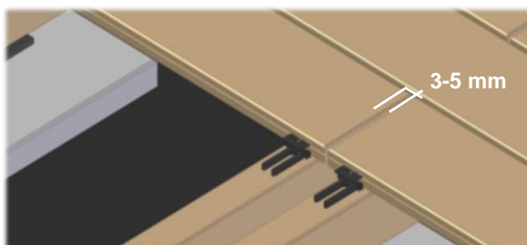
Figur 9: Skarvning av brädor över dubbla bjälkar.
